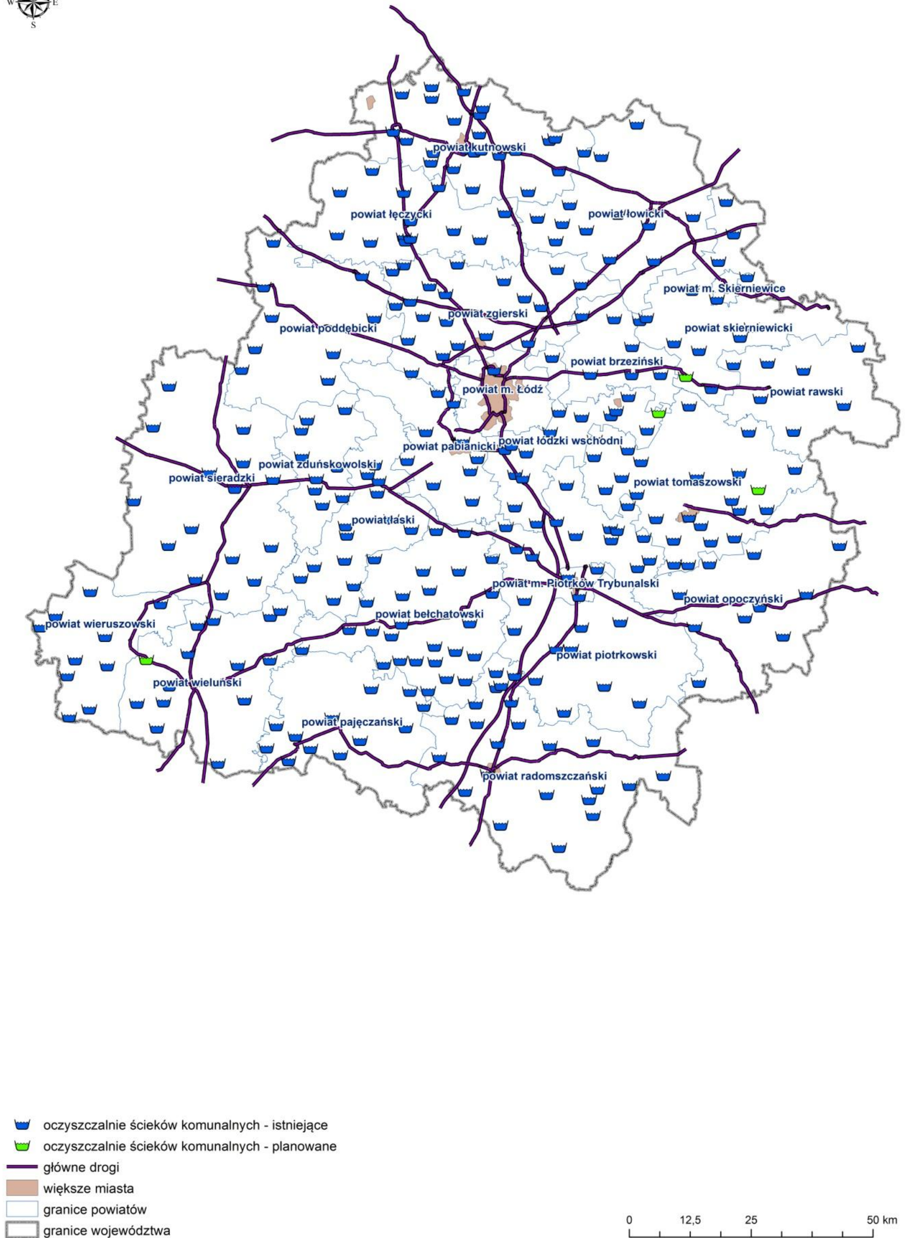
Rysunek 27. Lokalizacja komunalnych oczyszczalni ścieków - istniejących i planowanych 97
