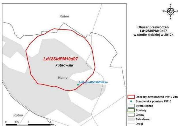
Źródło: Opracowanie B.S.I.P.P „EKOMETRIA” Sp. z o.o. Rys. 9. Obszar przekroczeń Ld12SidPM10d07 w strefie łódzkiej w 2012 r.
