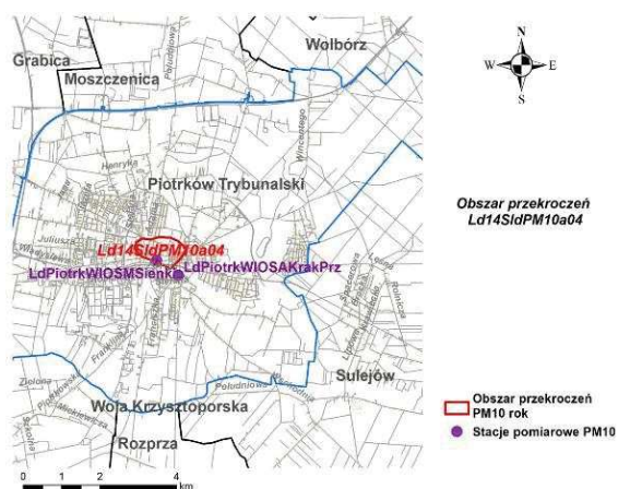
Rys. 89. Obszar przekroczeń Ld14SidPM10a04 w strefie łódzkiej w 2014 r.
