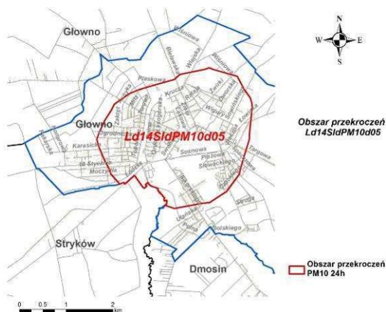
Rys. 21. Obszar przekroczeń Ld14SidPM10d05 w strefie łódzkiej w 2014 r.
