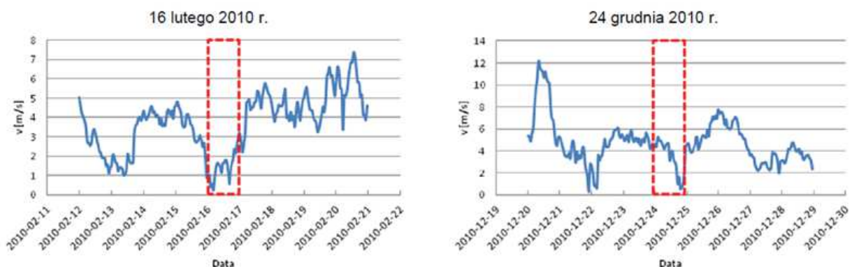
Rys. 74. Jednogodzinne wartości prędkości wiatru [m/s] dla wybranych dni na stanowisku w Kutnie, przy ul. Wilczej
