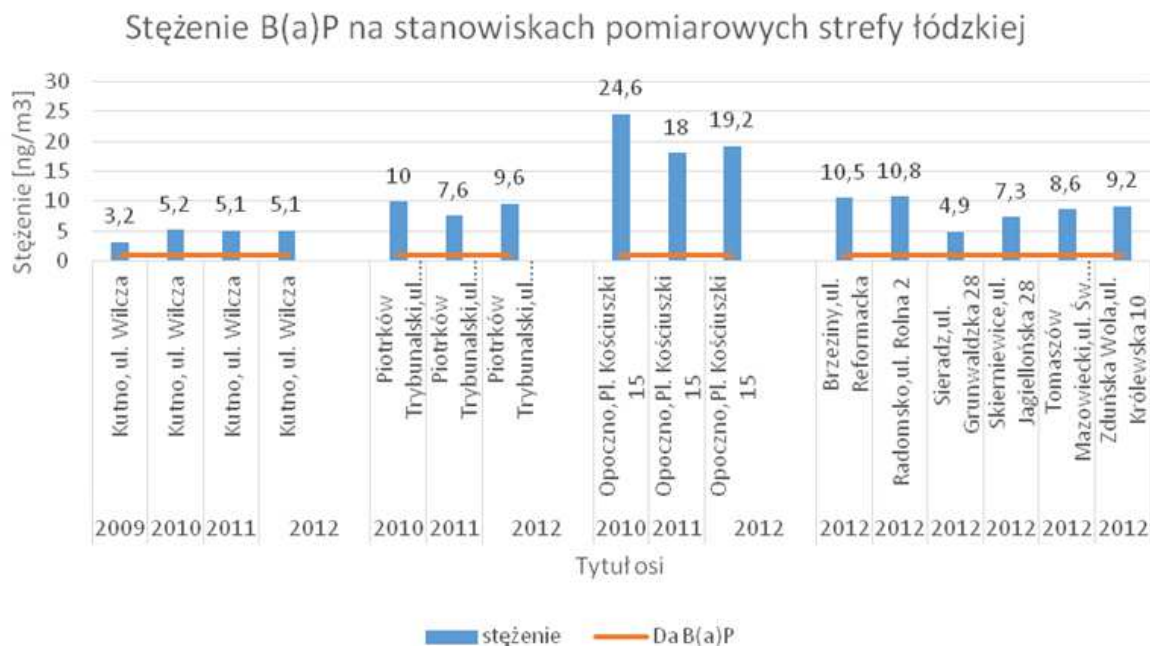
Rys. 51. Wyniki pomiarów stężeń benzo(a)pirenu w latach 2009 -2012 ze stanowisk pomiarowych z wojewódzkiej sieci monitoringu jakości powietrza WIOŚ w Łodzi.
