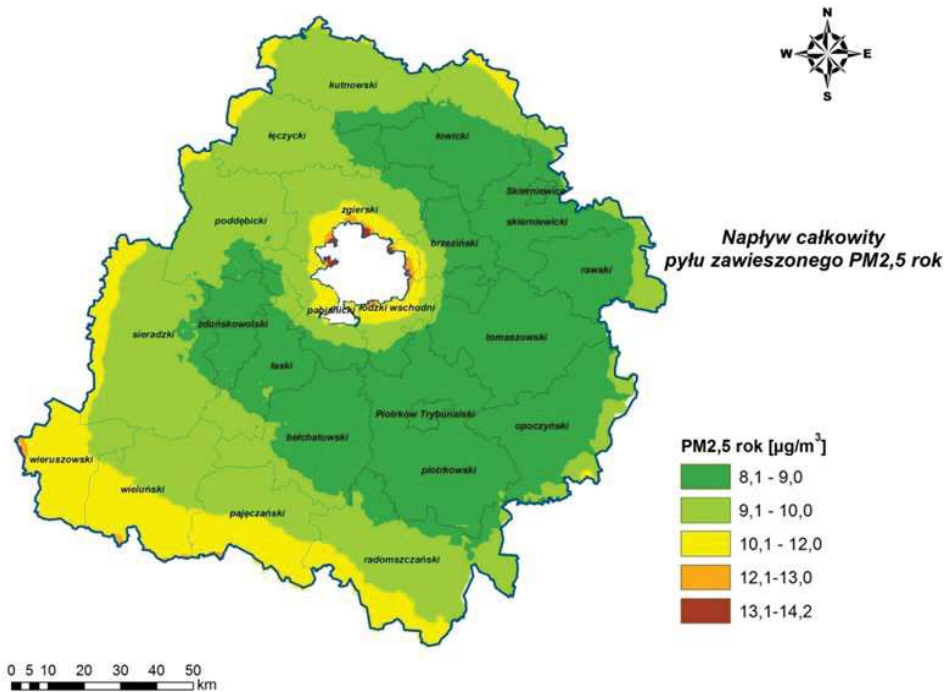
Rys. 35. Stężenia pyłu zawieszonego PM 2,5 o okresie uśredniania wyników rok kalendarzowy w strefie łódzkiej pochodzące z tła całkowitego w 2014 r.
