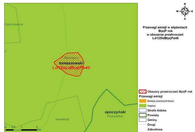
Rys. 203. Przewagi emisji w stężeniach B(a)P zawartego w pyłe zawieszonym PM10 w obszarze przekroczeń Ld12SIdB(a)Pa40 w strefie łódzkiej w 2012 r.”
