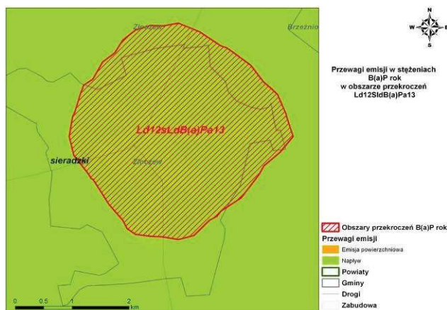
Rys. 151. Przewagi emisji w stężeniach B(a)P zawartego w pyłe zawieszonym PM10 w obszarze przekroczeń Ld12SldB(a)Pa13 w strefie łódzkiej w 2012 r.
