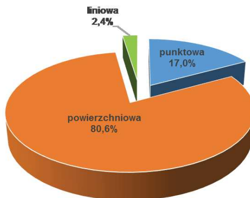
Rys. 33. Udział procentowy emisji B(a)P poszczególnych typów ze strefy łódzkiej w 2014 r.
