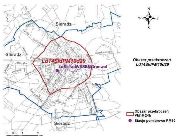
Rys. 61. Obszar przekroczeń Ld14SidPM10d29 w strefie łódzkiej w 2014 r.
