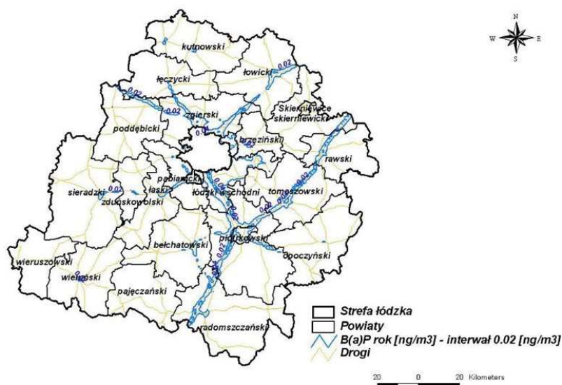
Rys. 66. Stężenia B(a)P o okresie uśredniania wyników rok kalendarzowy w strefie łódzkiej pochodzące z emisji liniowej w 2011 r.
