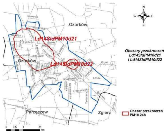
Rys. 49. Obszary przekroczeń Ld14SidPM10d21 i Ld14SidPM10d22 w strefie łódzkiej w 2014 r.
