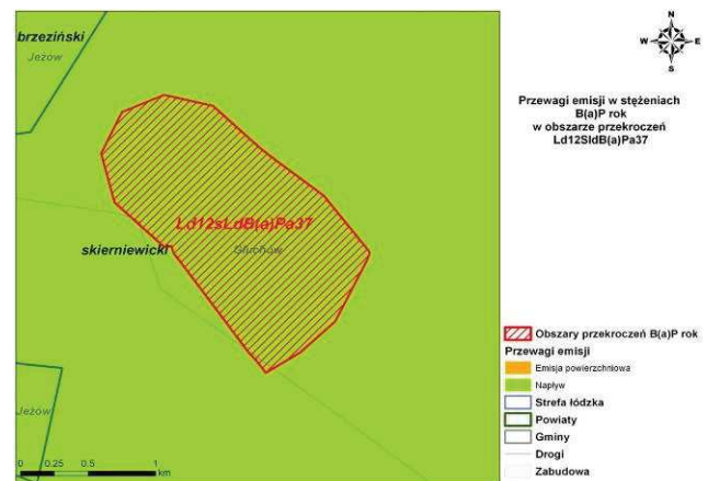
Rys. 199. Przewagi emisji w stężeniach B(a)P zawartego w pyłe zawieszonym PM10 w obszarze przekroczeń Ld12SldB(a)Pa37 w strefie łódzkiej w 2012 r.
