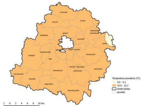
Rys. 44. Rozkład średniej rocznej temperatury powietrza [°C] wyznaczony przez model WRF/CALMET w strefie łódzkiej w 2014 r.
