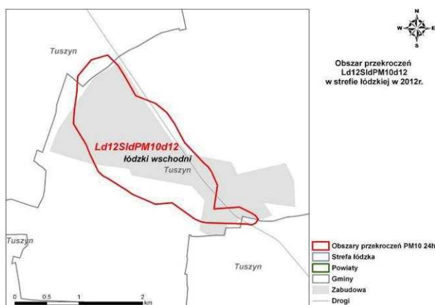
Źródło: Opracowanie B.S.I.P.P „EKOMETRIA” Sp. z o.o. Rys. 11. Obszar przekroczeń Ld12SidPM10d12 w strefie łódzkiej w 2012 r.
