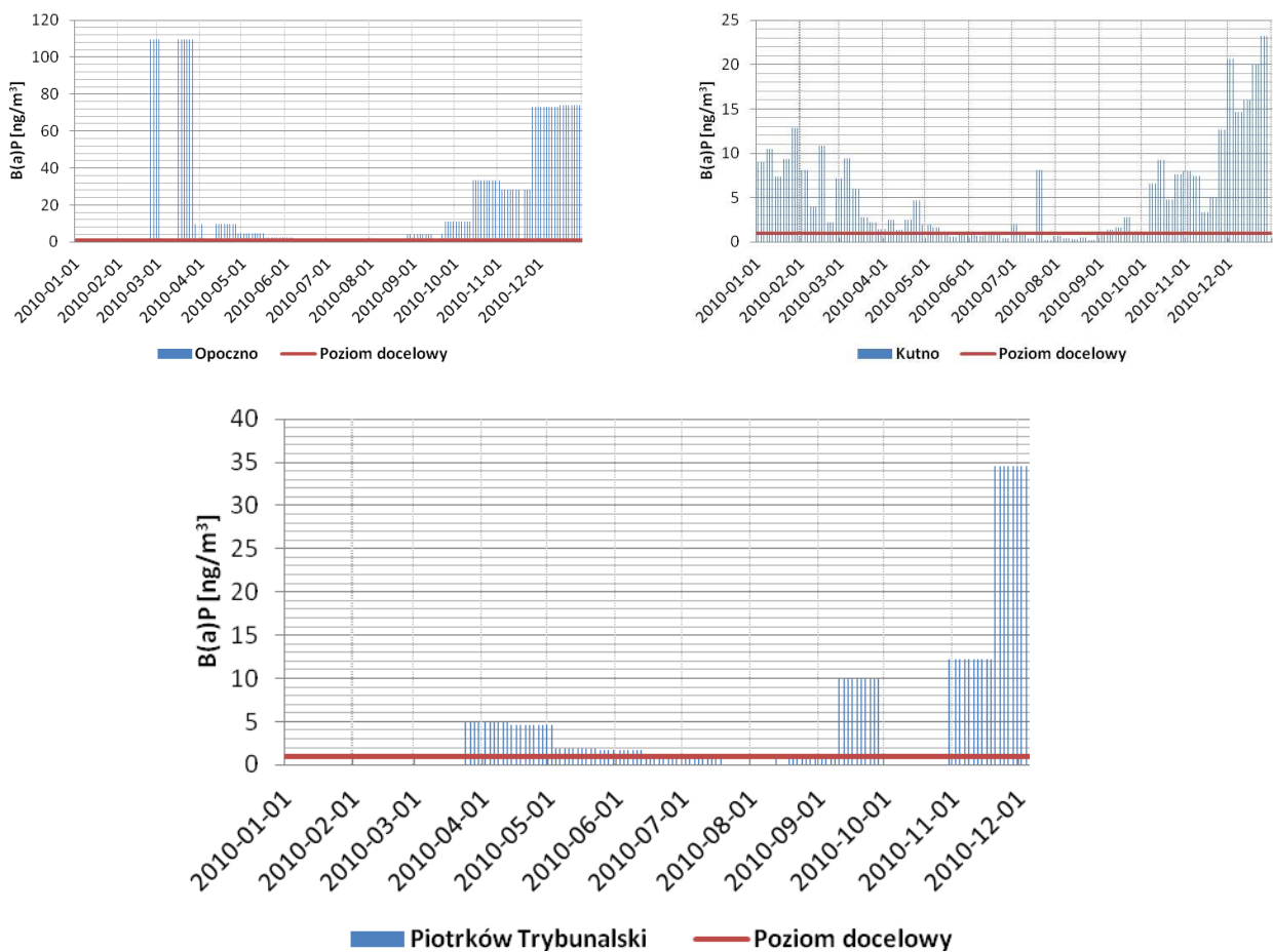
Rys. 52. Roczny przebieg średnich dobowych wartości B(a)P na wybranych stanowiskach pomiarowych w strefy łódzkiej w 2010 r.
