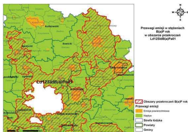
Rys. 125. Przewagi emisji w stężeniach B(a)P zawartego w pyłe zawieszonym PM10 w obszarze przekroczeń Ld12SIdB(a)Pa01 w strefie łódzkiej w 2012 r. – część 1
