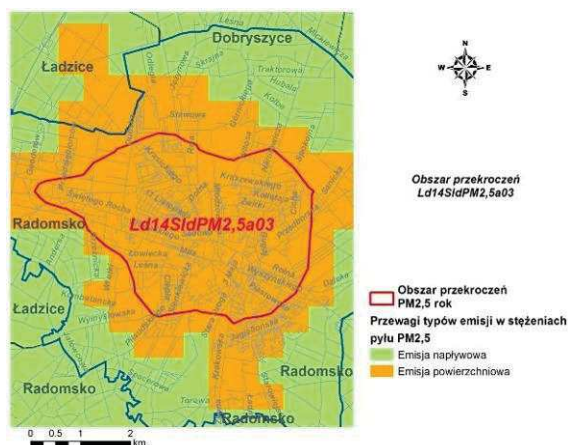
Źródło: Opracowanie B.S.I.P.P „EKOMETRIA” Sp. z o.o. Rys. 102. Przewagi typów emisji w obszarze przekroczeń Ld14SidPM2,5a03 w strefie łódzkiej w 2014 r.
