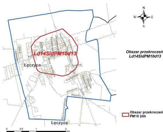
Rys. 37. Obszar przekroczeń Ld14SidPM10d13 w strefie łódzkiej w 2014 r.
