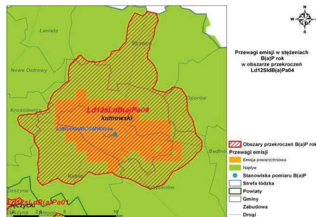
Źródło: Opracowanie B.S.I.P.P. „EKOMETRIA” Sp. z o.o. Rys. 133. Przewagi emisji w stężeniach B(a)P zawartego w pyle zawieszonym PM10 w obszarze przekroczeń Ld12SIdB(a)Pa04 w strefie łódzkiej w 2012 r.
