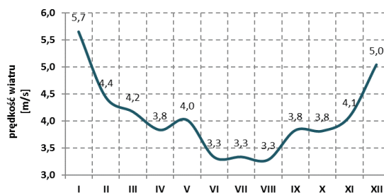
Źródło: Opracowanie B.S.I.P.P. „EKOMETRIA” Sp. z o.o. Rys. 19. Średnia miesięczna prędkość wiatru [m/s] wyznaczona przez model WRF/CALMET w strefie łódzkiej w 2014 r.
