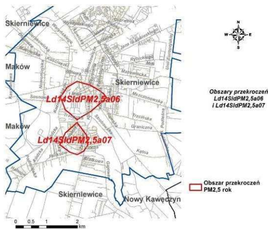
Rys. 107. Obszary przekroczeń Ld14SidPM2,5a06 i Ld14SidPM2,5a07 w strefie łódzkiej w 2014 r.
