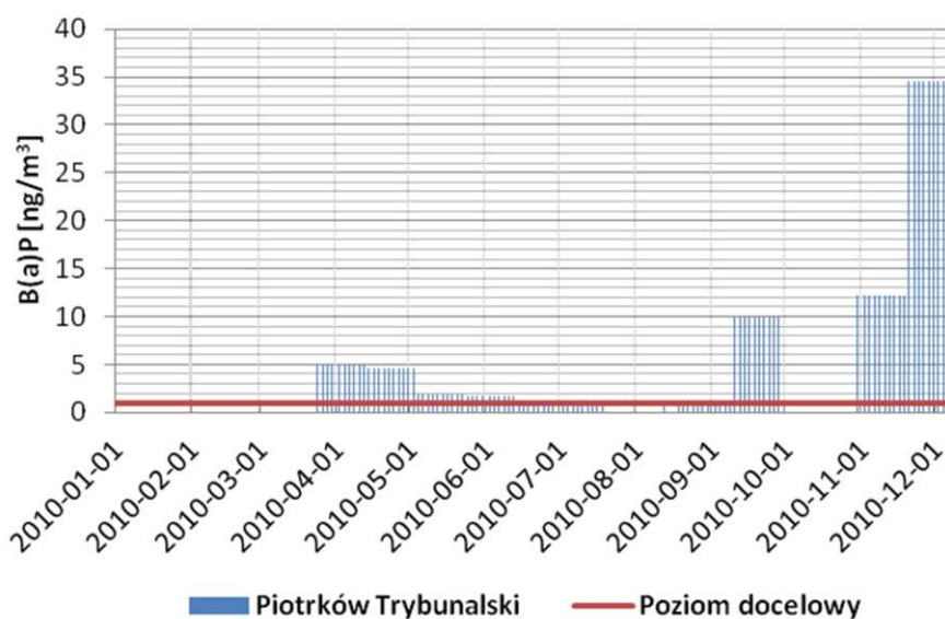
Rys.13. Roczny przebieg średniodobowych wartości stężeń benzo(a)pirenu zawartego w pyłe zawieszonym PM10 na stanowisku pomiarowym w Piotrkowie Trybunalskim przy ul. Sienkiewicza w 2010 roku.
