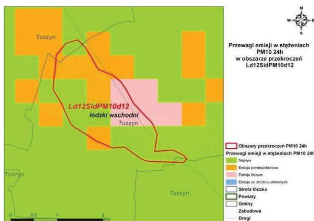
Źródło: Opracowanie B.S.I.P.P „EKOMETRIA” Sp. z o.o. Rys. 12. Przewagi typów emisji w obszarze przekroczeń Ld12SidPM10d12 w strefie łódzkiej w 2012 r.
