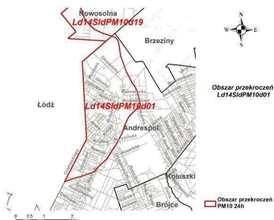
Rys. 13. Obszar przekroczeń Ld14SidPM10d01 w strefie łódzkiej w 2014 r.
