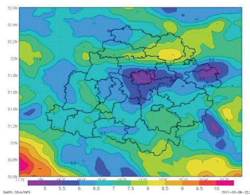
Rys.2. Przestrzenny rozkład częstości występowania cisz atmosferycznych ( v < 1,5[m/s] ) wyznaczonych przez model WRF/CALMET dla strefy łódzkiej w 2010 r.
