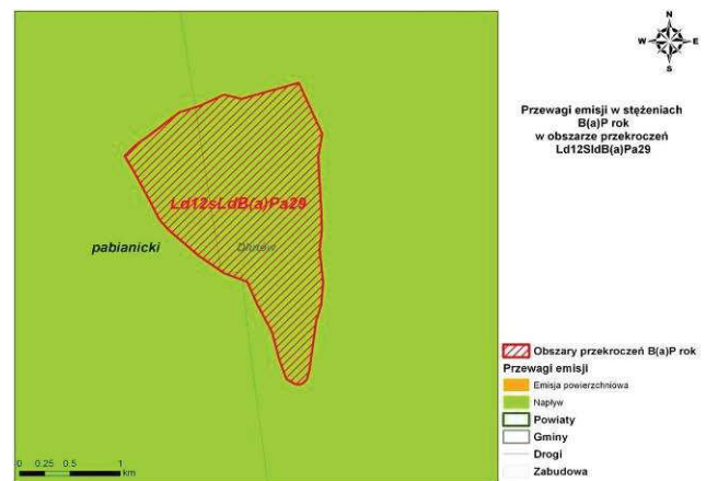
Rys. 183. Przewagi emisji w stężeniach B(a)P zawartego w pyłe zawieszonym PM10 w obszarze przekroczeń Ld12SldB(a)Pa29 w strefie łódzkiej w 2012 r.
