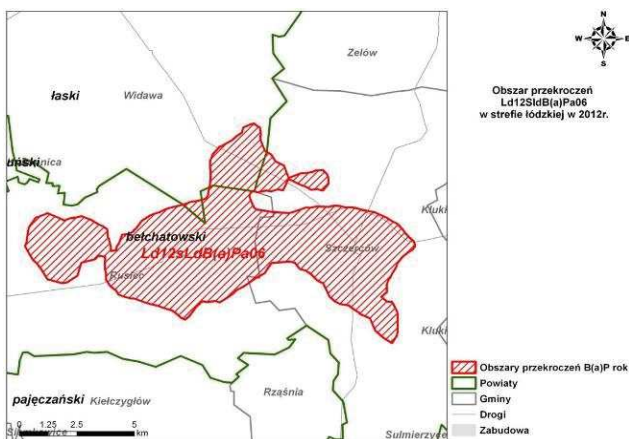
Rys. 136. Obszar przekroczeń Ld12SIdB(a)Pa06 w strefie łódzkiej w 2012 r.
