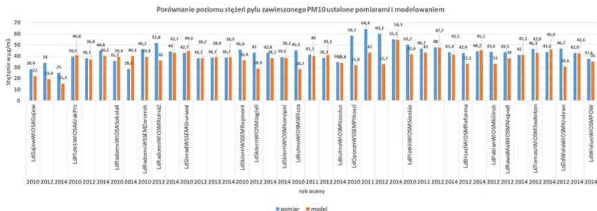
Rys. 10. Zestawienie poziomu stężeń pyłu zawieszonego PM10 wyznaczonych pomiarami ze stężeniami pyłu zawieszonego PM10 wyznaczonymi na podstawie modelowania
