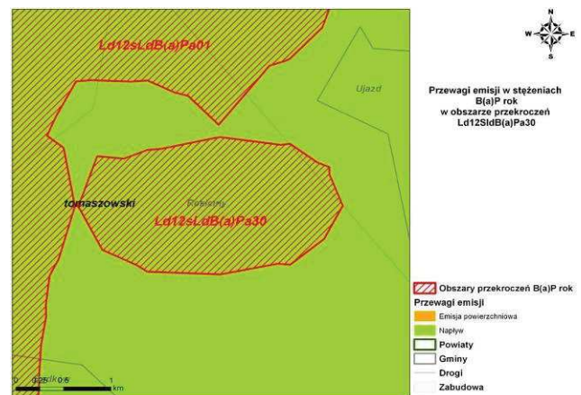
Rys. 185. Przewagi emisji w stężeniach B(a)P zawartego w pyłe zawieszonym PM10 w obszarze przekroczeń Ld12SldB(a)Pa30 w strefie łódzkiej w 2012 r.
