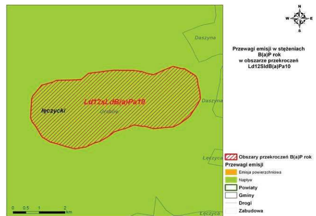
Rys. 145. Przewagi emisji w stężeniach B(a)P zawartego w pyłe zawieszonym PM10 w obszarze przekroczeń Ld12SldB(a)Pa10 w strefie łódzkiej w 2012 r.
