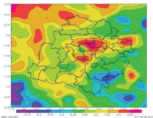
Rys.1. Przestrzenny rozkład średnich rocznych wartości prędkości wiatru wyznaczonych przez model WRF/CALMET w strefie łódzkiej w 2010 r.
