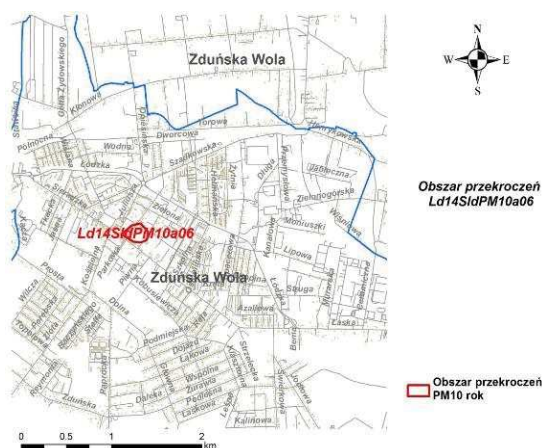
Rys. 93. Obszar przekroczeń Ld14SidPM10a06 w strefie łódzkiej w 2014 r.
