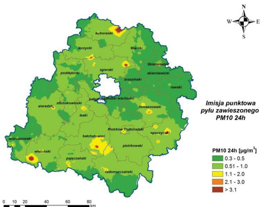
Rys. 36. Stężenia pyłu zawieszonego PM10 o okresie uśredniania wyników 24 godziny w strefie łódzkiej pochodzące z emisji punktowej w 2014 r.
