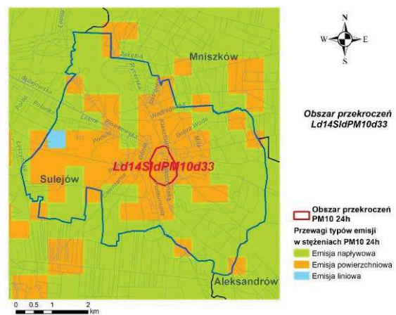
Rys. 68. Przewagi typów emisji w obszarze przekroczeń Ld14SidPM10d33 w strefie łódzkiej w 2014 r.
