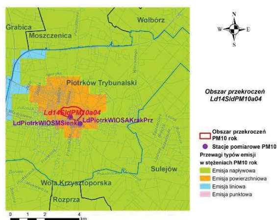
Rys. 90. Przewagi typów emisji w obszarze przekroczeń Ld14SidPM10a04 w strefie łódzkiej w 2014 r.
