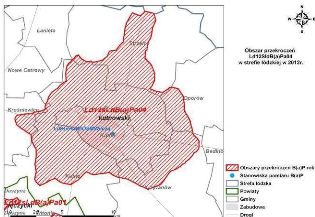
Źródło: Opracowanie B.S.I.P.P. „EKOMETRIA” Sp. z o.o. Rys. 132. Obszar przekroczeń Ld12SIdB(a)Pa04 w strefie łódzkiej w 2012 r.
