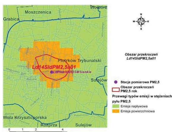
Źródło: Opracowanie B.S.I.P.P. „EKOMETRIA” Sp. z o.o. Rys. 98. Przewagi typów emisji w obszarze przekroczeń Ld14SidPM2,5a01 w strefie łódzkiej w 2014 r.
