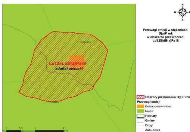
Rys. 161. Przewagi emisji w stężeniach B(a)P zawartego w pyłe zawieszonym PM10 w obszarze przekroczeń Ld12SIdB(a)Pa18 w strefie łódzkiej w 2012 r.
