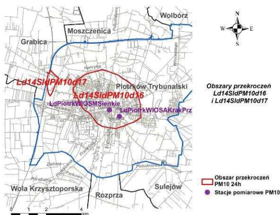
Rys. 41. Obszary przekroczeń Ld14SidPM10d16 i Ld14SidPM10d17 w strefie łódzkiej w 2014 r.
