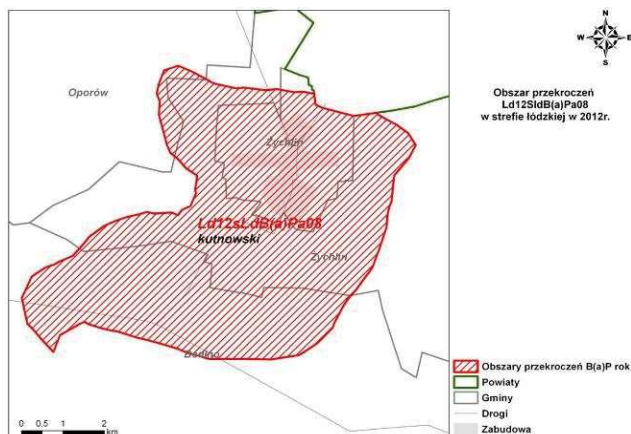
Rys. 140. Obszar przekroczeń Ld12SIdB(a)Pa08 w strefie łódzkiej w 2012 r.
