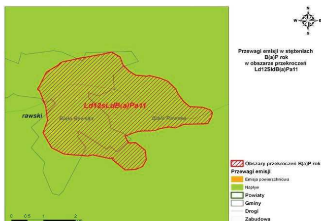
Rys. 147. Przewagi emisji w stężeniach B(a)P zawartego w pyłe zawieszonym PM10 w obszarze przekroczeń Ld12SIdB(a)Pa11 w strefie łódzkiej w 2012 r.
