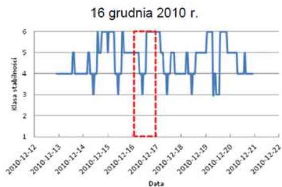
Rys. 16. Klasy równowagi atmosfery dla wybranych dni na stanowisku w Opocznie, Plac Kościuszki
