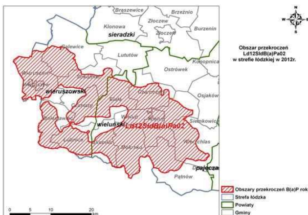
Rys. 128. Obszar przekroczeń Ld12SIdB(a)Pa02 w strefie łódzkiej w 2012 r.
