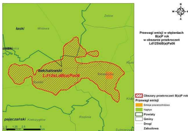
Rys. 137. Przewagi emisji w stężeniach B(a)P zawartego w pyłe zawieszonym PM10 w obszarze przekroczeń Ld12SIdB(a)Pa06 w strefie łódzkiej w 2012 r.
