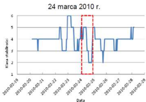
Rys. 16. Klasy równowagi atmosfery dla wybranych dni na stanowisku w Opocznie, Plac Kościuszki
