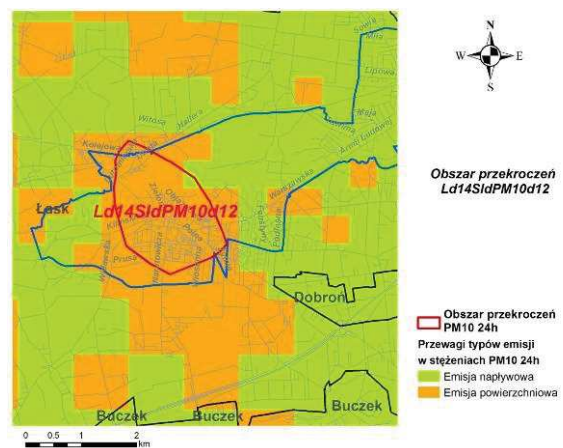
Źródło: Opracowanie B.S.I.P.P „EKOMETRIA” Sp. z o.o. Rys. 36. Przewagi typów emisji w obszarze przekroczeń Ld14SidPM10d12 w strefie łódzkiej w 2014 r.
