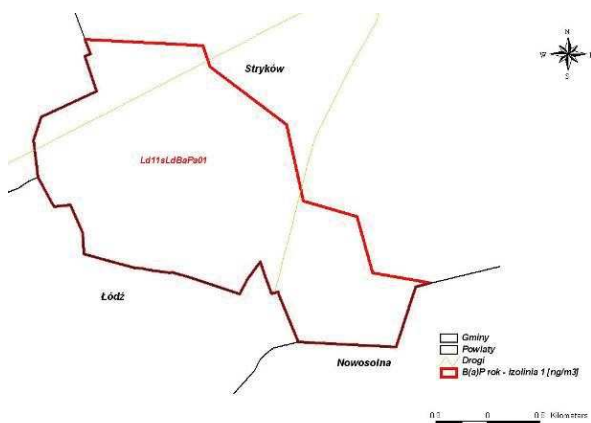
Źródło: Opracowanie B.S.I.P.P „EKOMETRIA” Sp. z o.o. Rys. 116. Obszar przekroczeń Ld11SldB(a)Pa01 w strefie łódzkiej w 2011 r.
