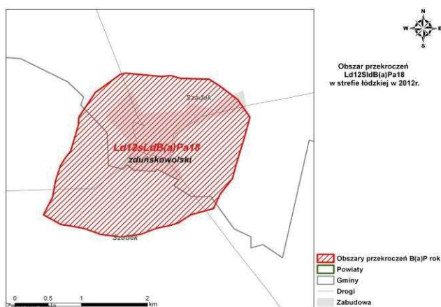
Rys. 160. Obszar przekroczeń Ld12SIdB(a)Pa18 w strefie łódzkiej w 2012 r.
