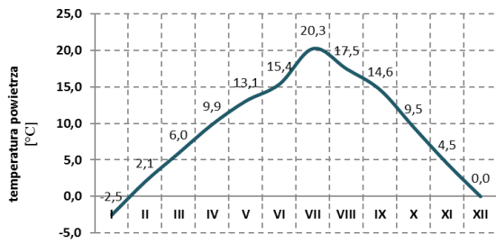
Rys. 43. Przebieg średnich miesięcznych wartości temperatury powietrza wyznaczonych przez model WRF/CALMET w strefie łódzkiej w 2014 r.
