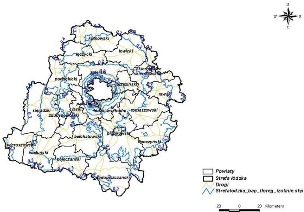
Rys. 62. Stężenia B(a)P o okresie uśredniania wyników rok kalendarzowy w strefie łódzkiej pochodzące z tła regionalnego w 2011 r.
