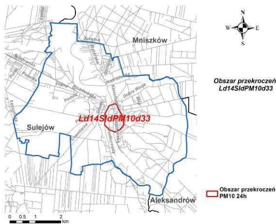
Rys. 67. Obszar przekroczeń Ld14SidPM10d33 w strefie łódzkiej w 2014 r.
