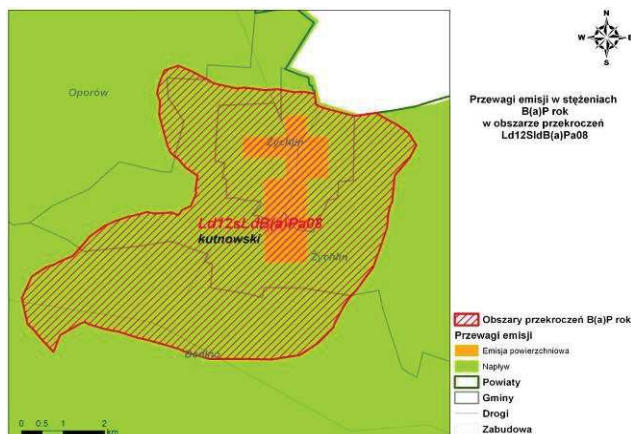
Rys. 141. Przewagi emisji w stężeniach B(a)P zawartego w pyłe zawieszonym PM10 w obszarze przekroczeń Ld12SIdB(a)Pa08 w strefie łódzkiej w 2012 r.
