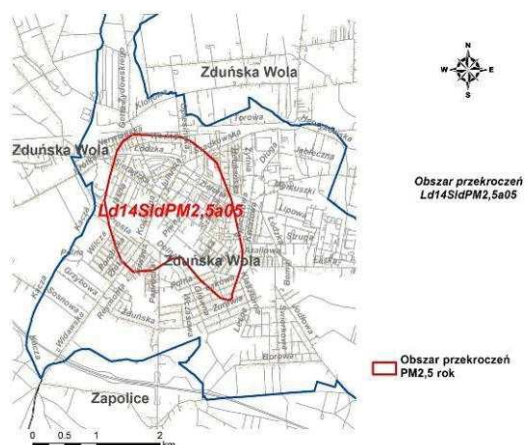
Rys. 105. Obszar przekroczeń Ld14SidPM2,5a05 w strefie łódzkiej w 2014 r.
