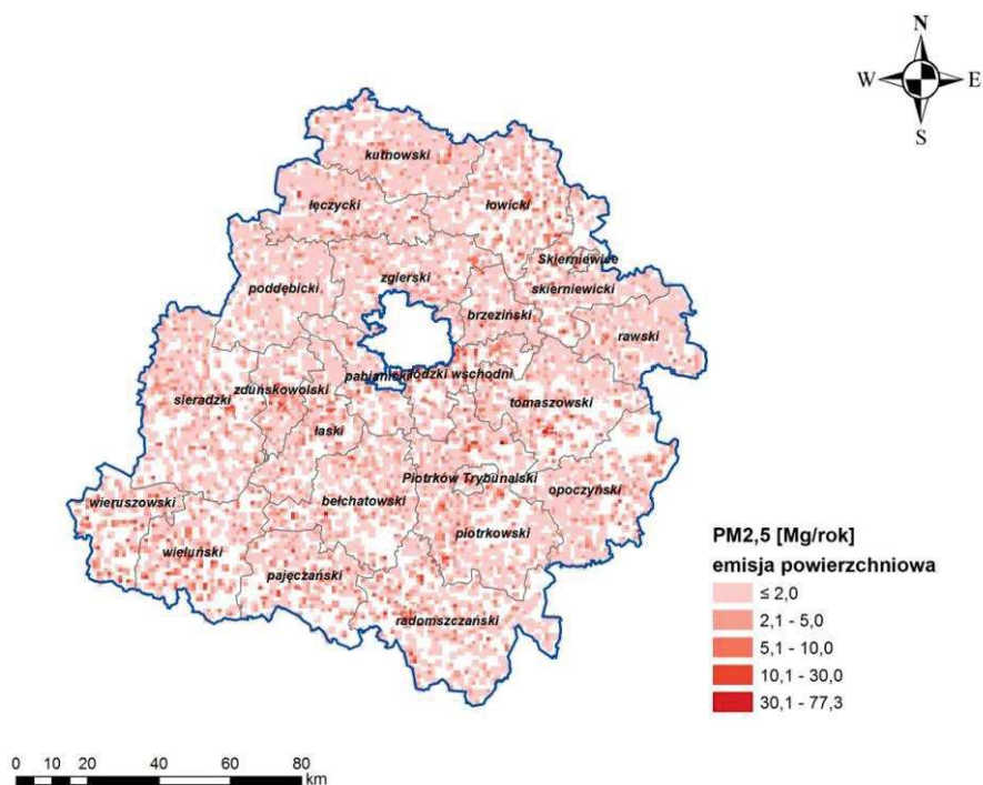
Rys. 11. Emisja powierzchniowa pyłu zawieszonego PM2,5 z terenu strefy łódzkiej w 2014 r.
