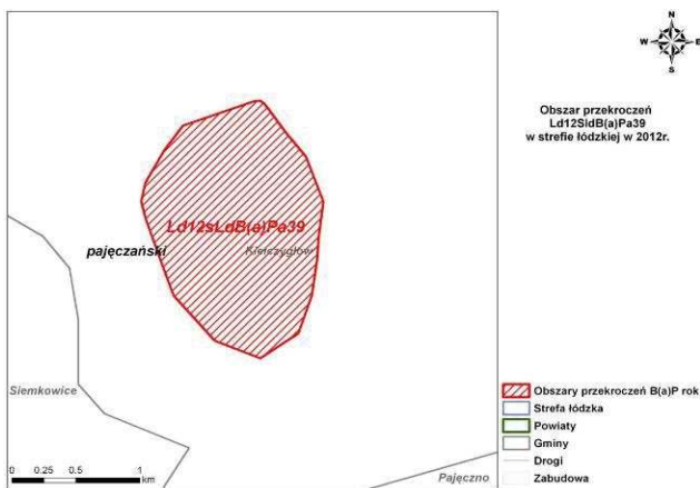
Rys. 200. Obszar przekroczeń Ld12SIdB(a)Pa39 w strefie łódzkiej w 2012 r.
