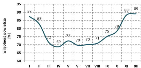
Rys. 38 Przebieg średnich miesięcznych wartości wilgotności względnej powietrza [%] wyznaczonej przez model WRF/CALMET w strefie łódzkiej w 2014 r.
