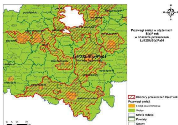
Rys. 127. Przewagi emisji w stężeniach B(a)P zawartego w pyłe zawieszonym PM10 w obszarze przekroczeń Ld12SIdB(a)Pa01 w strefie łódzkiej w 2012 r. – część 2
