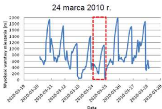
Rys. 17. Wysokość warstwy mieszania dla wybranych dni na stanowisku w Opocznie, Plac Kościuszki
