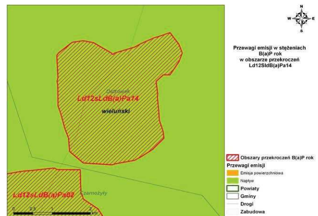
Rys. 153. Przewagi emisji w stężeniach B(a)P zawartego w pyłe zawieszonym PM10 w obszarze przekroczeń Ld12SldB(a)Pa14 w strefie łódzkiej w 2012 r.
