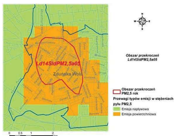
Rys. 106. Przewagi typów emisji w obszarze przekroczeń Ld14SidPM2,5a05 w strefie łódzkiej w 2014 r.
