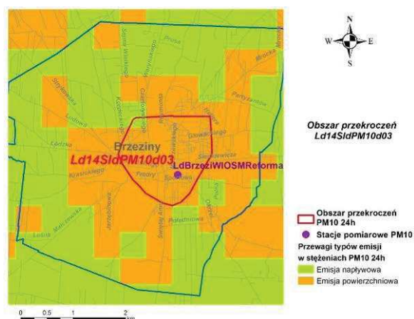
Źródło: Opracowanie B.S.I.P.P „EKOMETRIA” Sp. z o.o. Rys. 18. Przewagi typów emisji w obszarze przekroczeń Ld14SIdPM10d03 w strefie łódzkiej w 2014 r.
