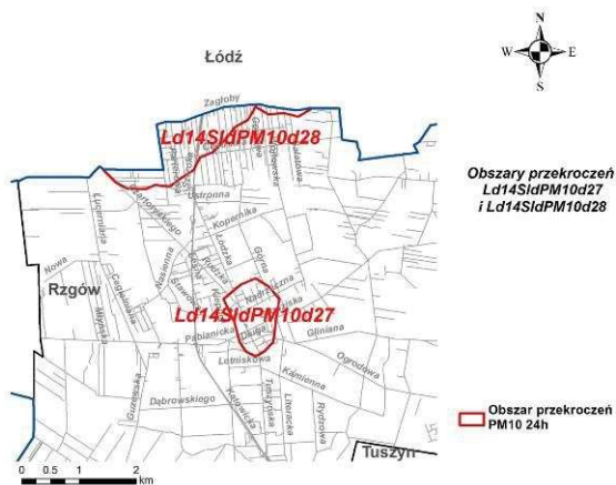
Rys. 59. Obszary przekroczeń Ld14SidPM10d27 i Ld14SidPM10d28 w strefie łódzkiej w 2014 r.
