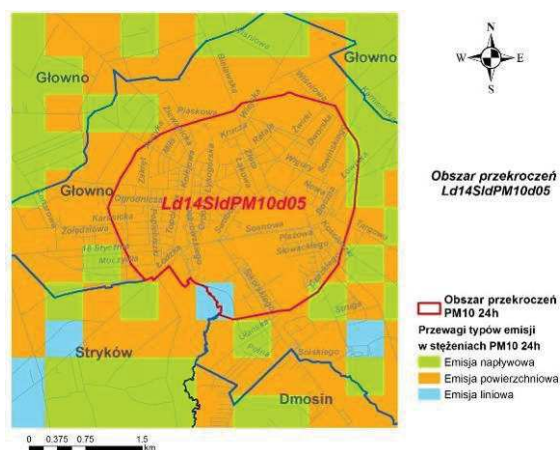
Rys. 22. Przewagi typów emisji w obszarze przekroczeń Ld14SidPM10d05 w strefie łódzkiej w 2014 r.
