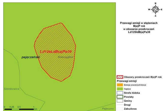
Rys. 201. Przewagi emisji w stężeniach B(a)P zawartego w pyłe zawieszonym PM10 w obszarze przekroczeń Ld12SIdB(a)Pa39 w strefie łódzkiej w 2012 r.
