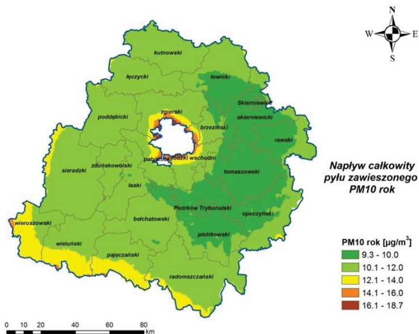
Rys. 34. Stężenia pyłu zawieszonego PM10 o okresie uśredniania wyników rok kalendarzowy w strefie łódzkiej pochodzące z tła całkowitego w 2014 r.
