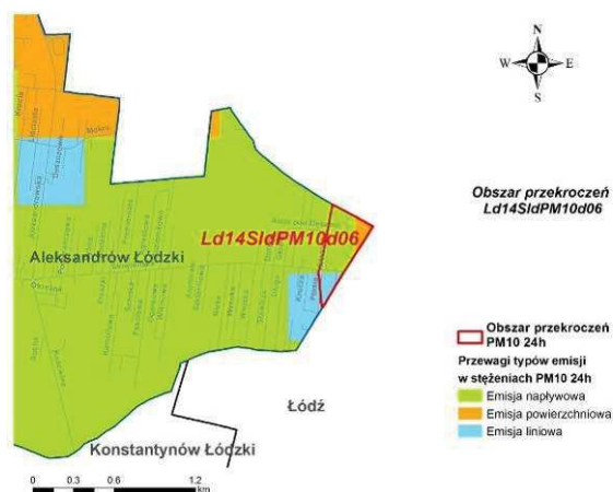
Rys. 24. Przewagi typów emisji w obszarze
