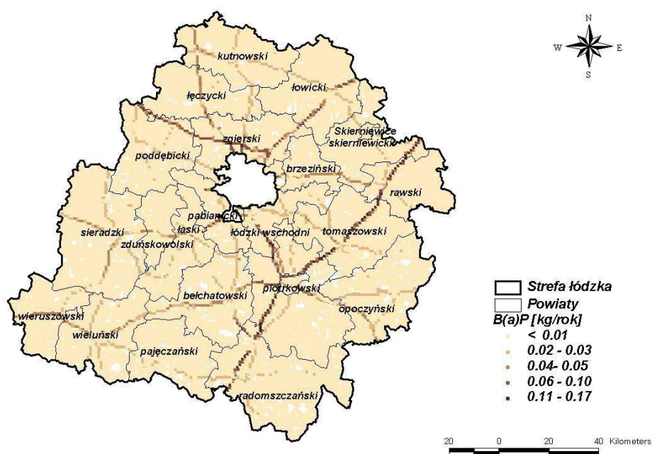
Rys. 28. Emisja liniowa B(a)P zawartego w pyłe zawieszonym PM10 z terenu strefy łódzkiej w 2011 r.
