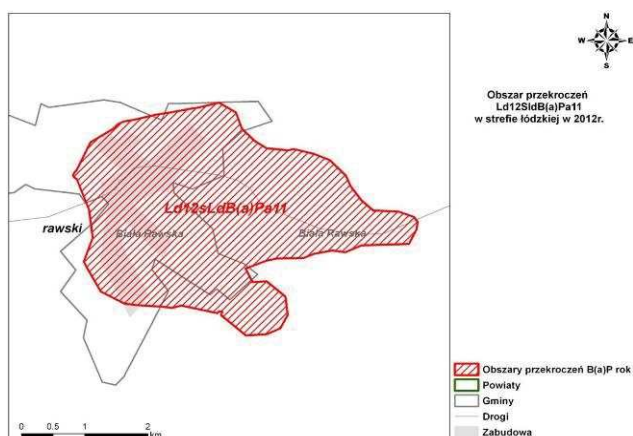
Rys. 146. Obszar przekroczeń Ld12SIdB(a)Pa11 w strefie łódzkiej w 2012 r.
