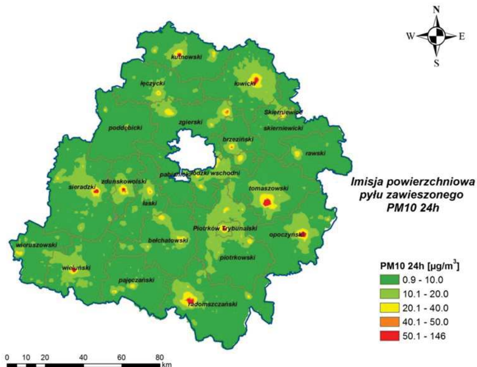
Rys. 38. Stężenia pyłu zawieszonego PM10 o okresie uśredniania wyników 24 godziny w strefie łódzkiej pochodzące z emisji powierzchniowej w 2014 r.
