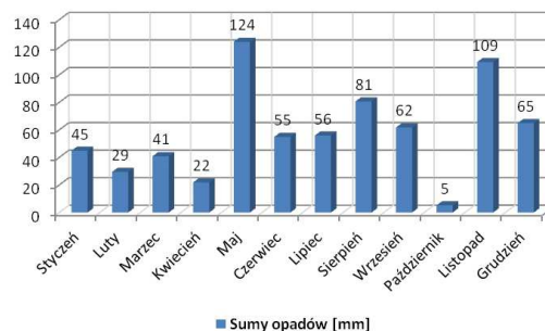
Rys. 26 Miesięczne sumy opadów atmosferycznych wyznaczone przez model WRF/CALMET w strefie łódzkiej w 2010 r.
