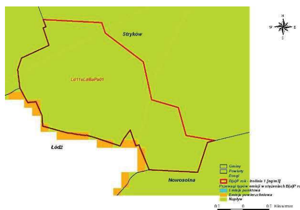
Źródło: Opracowanie B.S.I.P.P „EKOMETRIA” Sp. z o.o. Rys. 117. Przeważający typ emisji w stężeniach B(a)P zawartego w pyłe zawieszonym PM10, rok Ld11SldB(a)Pa01 w strefie łódzkiej w 2011 r.
