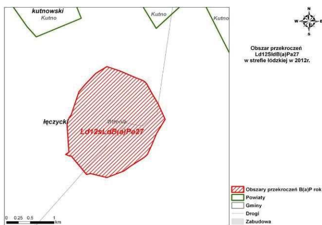
Rys. 178. Obszar przekroczeń Ld12SIdB(a)Pa27 w strefie łódzkiej w 2012 r.
