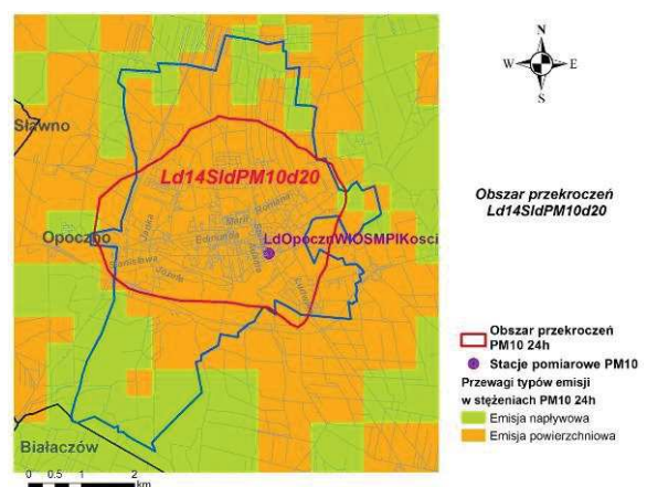
Źródło: Opracowanie B.S.I.P.P „EKOMETRIA” Sp. z o.o. Rys. 48. Przewagi typów emisji w obszarze przekroczeń Ld14SidPM10d20 w strefie łódzkiej w 2014 r.
