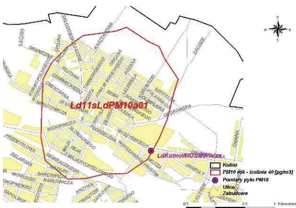
Źródło: Opracowanie B.S.I.P.P „EKOMETRIA” Sp. z o.o. Rys. 81. Obszar przekroczeń Ld11sLdPM10a01 w strefie łódzkiej w 2011 r.
