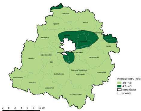
Źródło: Opracowanie B.S.I.P.P. „EKOMETRIA” Sp. z o.o. Rys.18. Rozkład średniej rocznej prędkości wiatru [m/s] wyznaczonej przez model WRF/CALMET w strefie łódzkiej w 2014 r.
