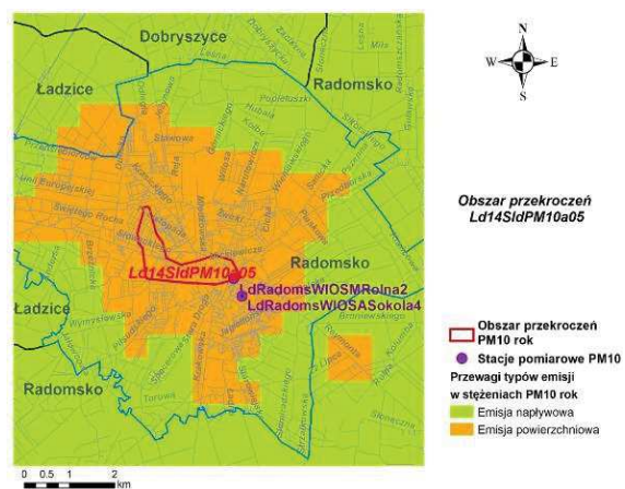
Źródło: Opracowanie B.S.I.P.P „EKOMETRIA” Sp. z o.o. Rys. 92. Przewagi typów emisji w obszarze przekroczeń Ld14SidPM10a05 w strefie łódzkiej w 2014 r.
