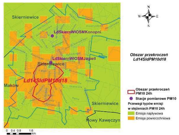
Rys. 44. Przewagi typów emisji w obszarze przekroczeń Ld14SidPM10d18 w strefie łódzkiej w 2014 r.
