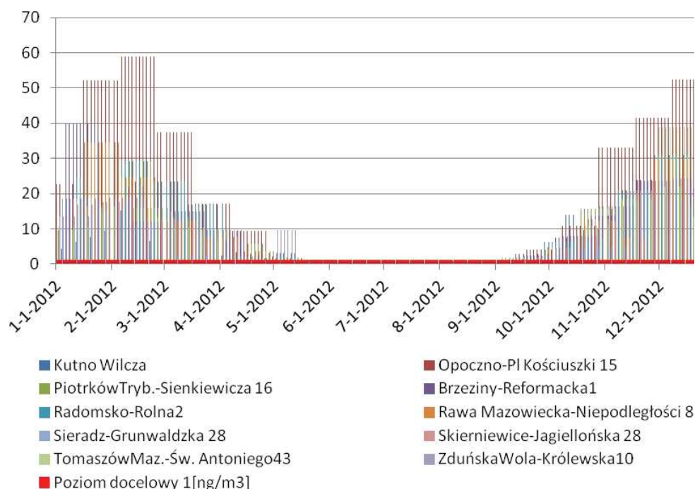
Rys. 15. Roczny przebieg średniodobowych wartości stężeń benzo(a)pirenu zawartego w pyłe zawieszonym PM10 na stanowiskach pomiarowych w strefie łódzkiej w 2012 roku.
