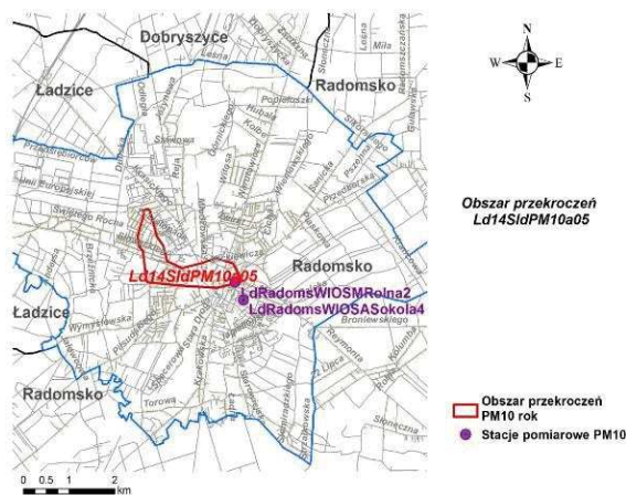
Źródło: Opracowanie B.S.I.P.P „EKOMETRIA” Sp. z o.o. Rys. 91. Obszar przekroczeń Ld14SidPM10a05 w strefie łódzkiej w 2014 r.
