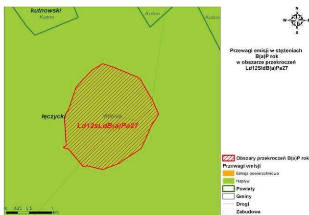
Rys. 179. Przewagi emisji w stężeniach B(a)P zawartego w pyłe zawieszonym PM10 w obszarze przekroczeń Ld12SIdB(a)Pa27 w strefie łódzkiej w 2012 r.
