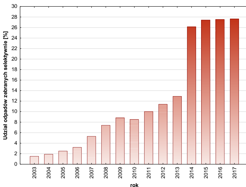
Rys. 9.2 Udział odpadów zebranych selektywnie w stosunku do ogółu odpadów w województwie łódzkim w latach 2003 – 2017 111
