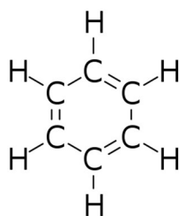
Rysunek 12. Struktura cząsteczki benzenu 17
