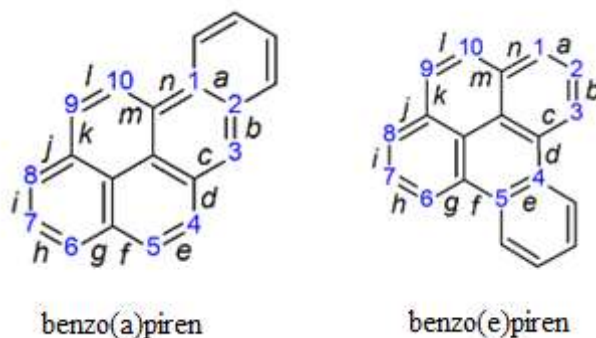
Rysunek 13. Porównanie cząsteczki benzo(a)pirenu oraz benzo(e)pirenu 18
